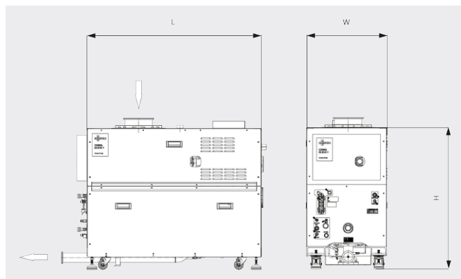
Dibujo dimensional
