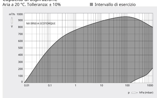
Capacità di aspirazione Aria a 20 °C. Tolleranza: \pm 10\%
