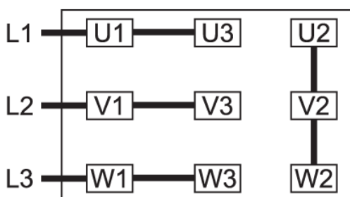
Collegamento a stella, motore multi-tensione con 9 pin (alta tensione):
