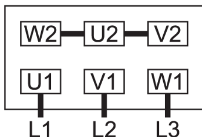
Collegamento a doppia stella, motore multi-tensione con 9 pin (bassa tensione):
