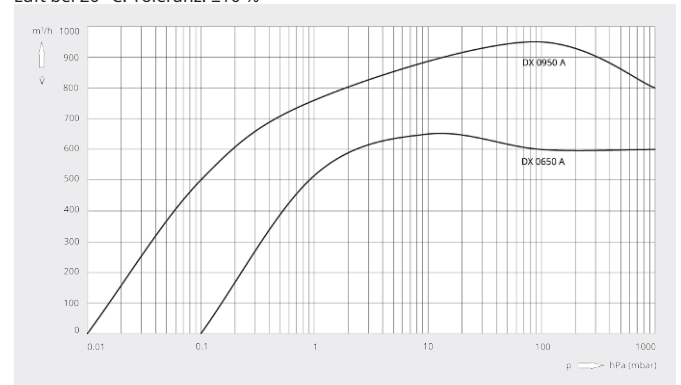
Saugvermögen Luft bei 20 °C. Toleranz: \pm 10\%
