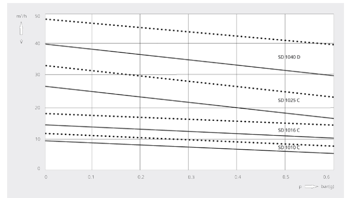
Volumenstrom
