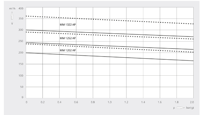
Débit volumétrique
