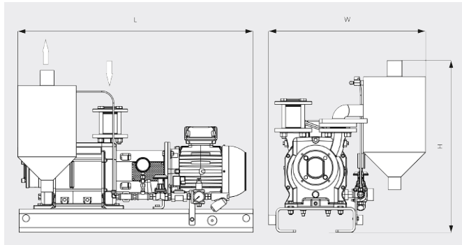
Maßzeichnung
