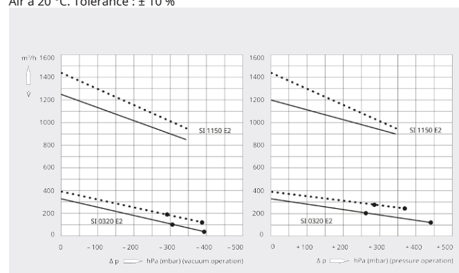
Vitesse de pompage/Débit volumétrique
