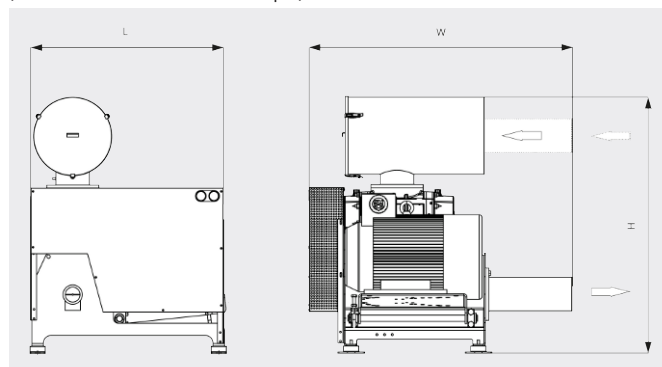
Schéma d'encombrement (sans caisson d'isolation acoustique)
