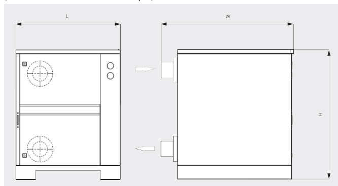
Schéma d'encombrement (avec caisson d'isolation acoustique)
