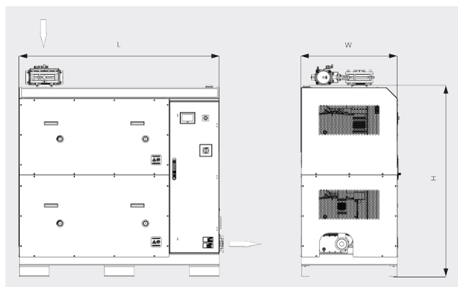
Dessin d'encombrement
