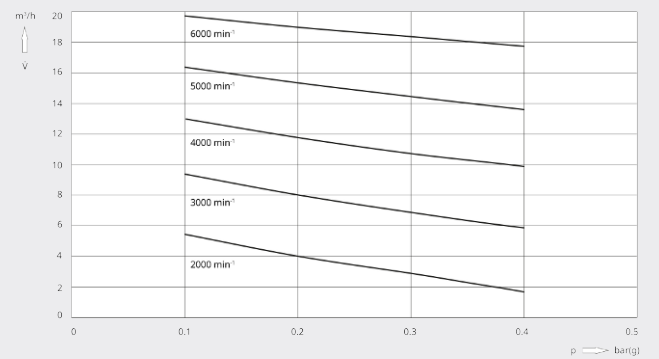
Saugvermögen
