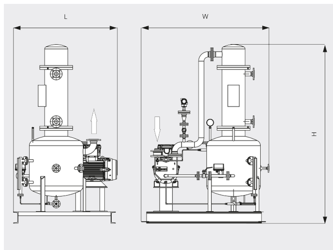
Dessin d'encombrement
