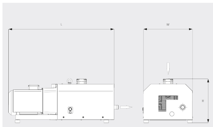
Dessin d'encombrement
