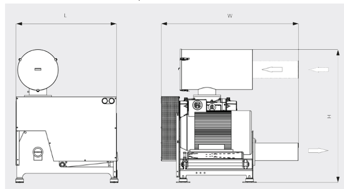
Dessin d'encombrement (sans caisson d'isolation acoustique)
