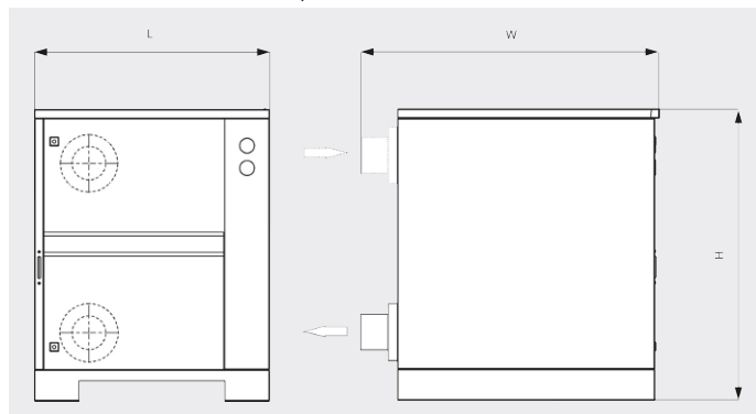
Dessin d'encombrement (avec caisson d'isolation acoustique)
