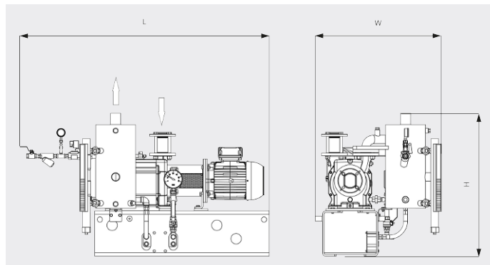
Dessin d'encombrement
