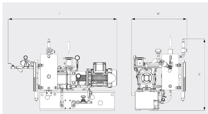
Dessin d'encombrement
