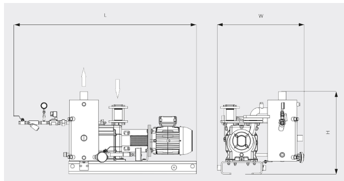
Dessin d'encombrement (zone sûre)
