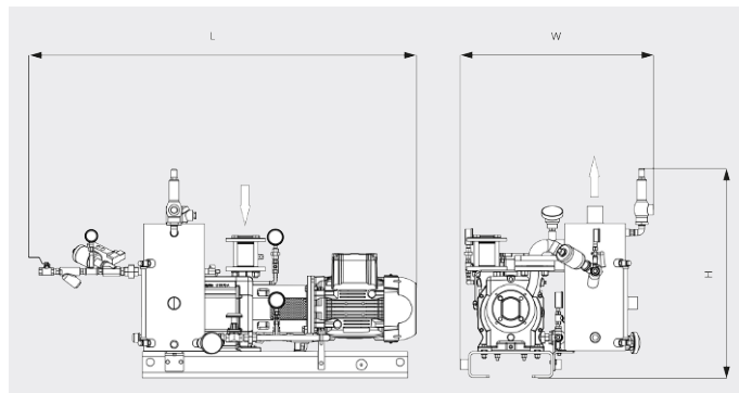
Dessin d'encombrement (en version ATEX)
