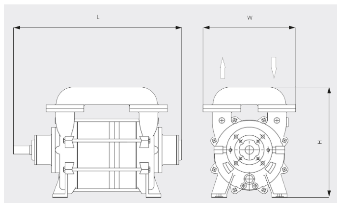
Dessin d'encombrement
