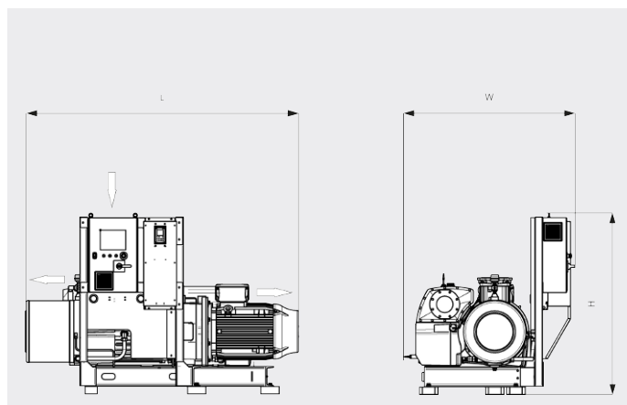
Dessin d'encombrement
