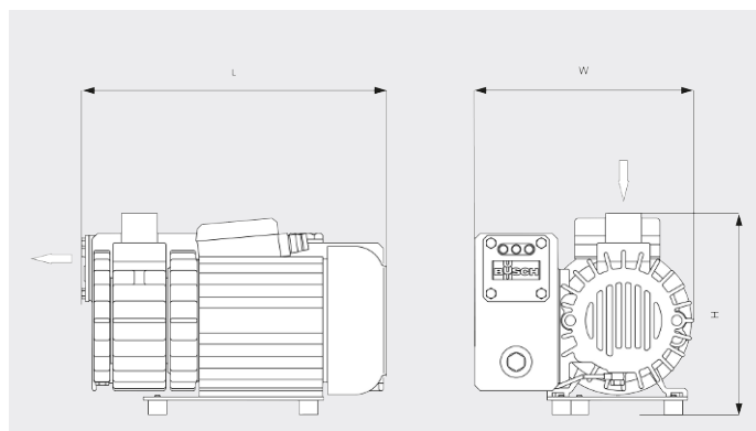
Dessin d'encombrement
