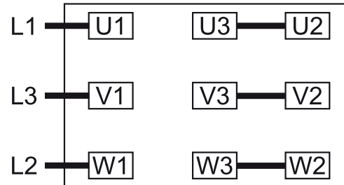
Steraansluiting, multispansingsmotor met 9 pinnen (hoogspanning):
