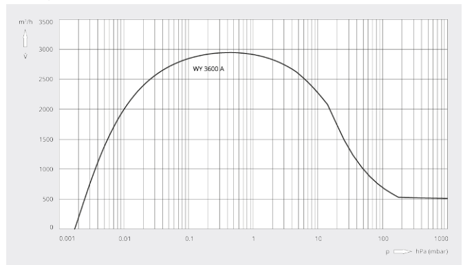
Pompsnelheid
