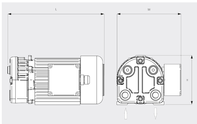
Dessin d'encombrement
