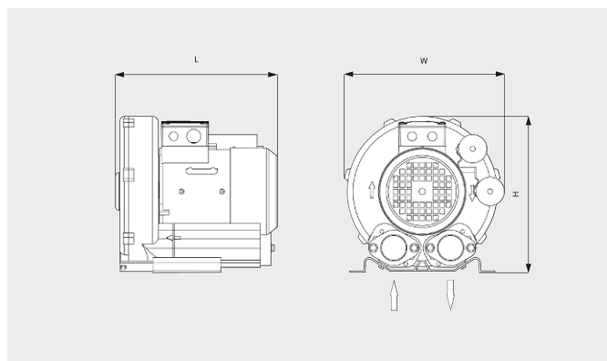
Maattekening
