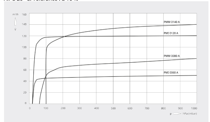
Vitesse de pompage Air à 20 °C. Tolérance : ± 10 %
