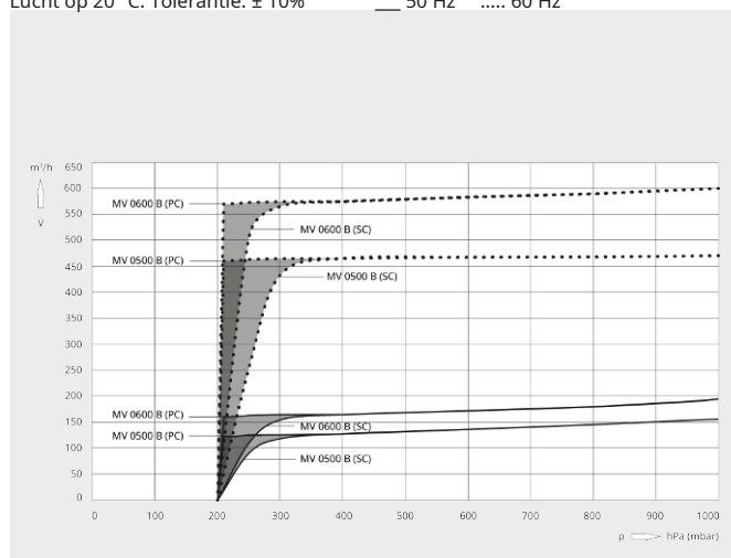
Pompsnelheid
