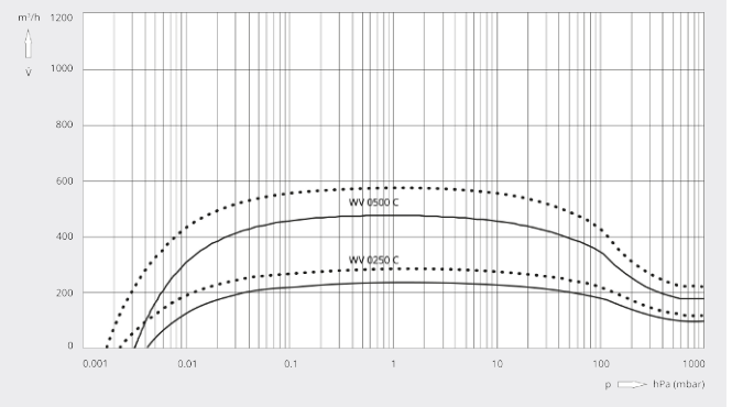
Pompsnelheid
