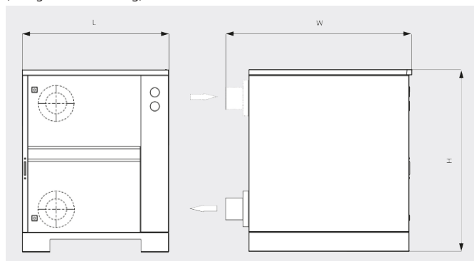
Maattekening (met geluidsomkasting)
