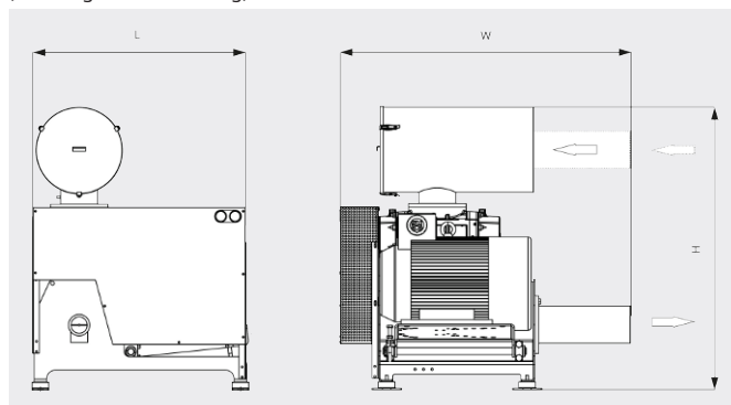
Maattekening (zonder geluidsomkasting)
