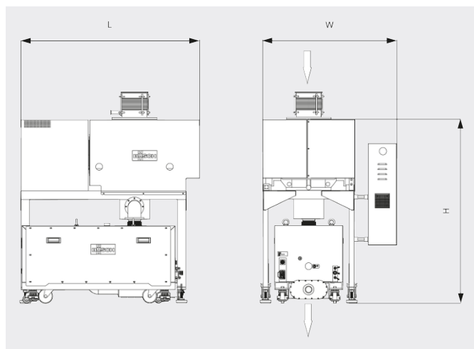
Dessin d'encombrement
