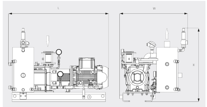
Maattekening
