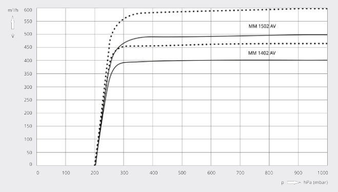
Pompsnelheid
