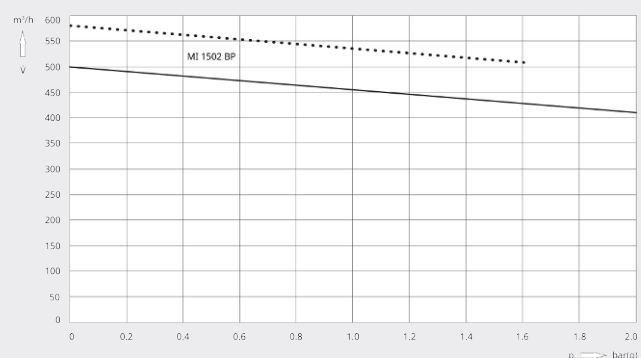
Vitesse de pompage Air à 20 °C. Tolérance : ± 10 %
