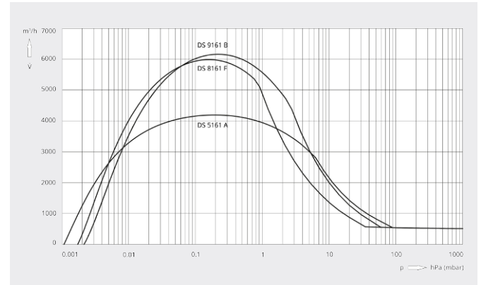
Vitesse de pompage Air à 20 °C. Tolérance : ± 10 %
