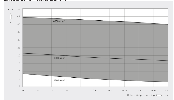
Volumenstrom (am Einlass) Luft bei 20 °C. Toleranz: \pm 10\%
