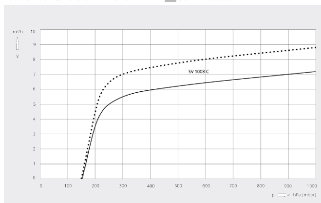
Saugvermögen
