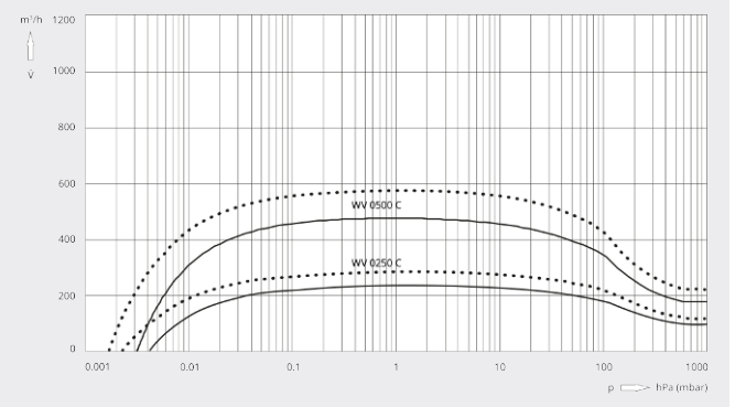
Saugvermögen
