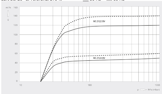
Saugvermögen
